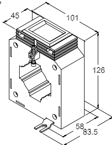
DIMENSIONS
