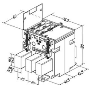
M3N1-25
